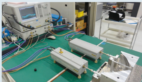
ミリ波帯誘電率測定システム
