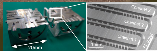
広帯域同時受信を目指した導波管フィルタ回路
