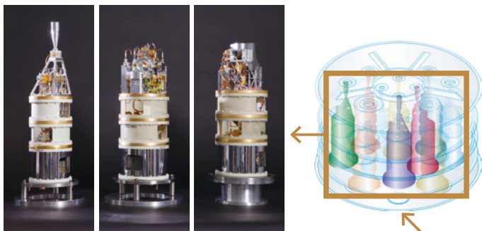
先端技術センターで開発したアルマ望遠鏡搭載受信機 左から Band4 (125-163GHz)、Band8 (385-500GHz)、 Band10 (787-950GHz) アルマ望遠鏡のアンテナは全部で 10種類の受信機を搭載する。
