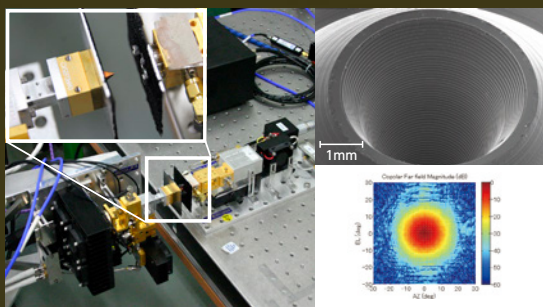
(左) 1.25-1.5THz帯コルゲートホーンの ビームパターン測定の様子
