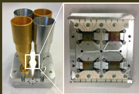
開発中の多素子集積型 SIS (超伝導体-絶縁体-超伝導体) 受信機
