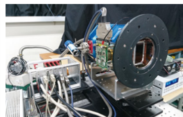
CCD 評価装置
