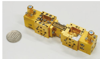
超低消費電力マイクロ波増幅器
