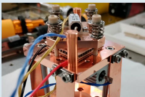
ペルチェ素子の低温評価試験
