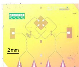
シリコン基板を用いた超伝導集積回路
