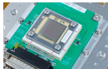
試験中の近赤外線検出器
