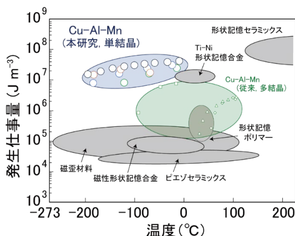
図 2. 温度と発生仕事量の関係。Cu-Al-Mn 合金は、従来の材料では実現できなかった -100^{\circ}\text{C} 以下の低温域での大きな仕事量を発生させることができる。
