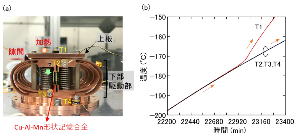
図 3. (a) 試作した機械式ヒートスイッチの外観。(b) 上板を加熱したときの T1～T4 における温度変化。
