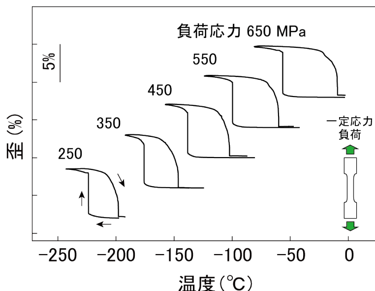
図 1. 一定応力下で冷却・加熱中の Cu-Al-Mn-Ni 形状記憶合金の歪みの変化。
